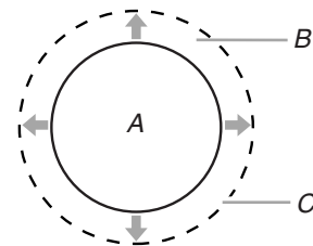
A. Surface de la zone de cuisson B. Ustensile de cuisson/autoclave C. Dépassement maximal de ½" (1,3 cm)
